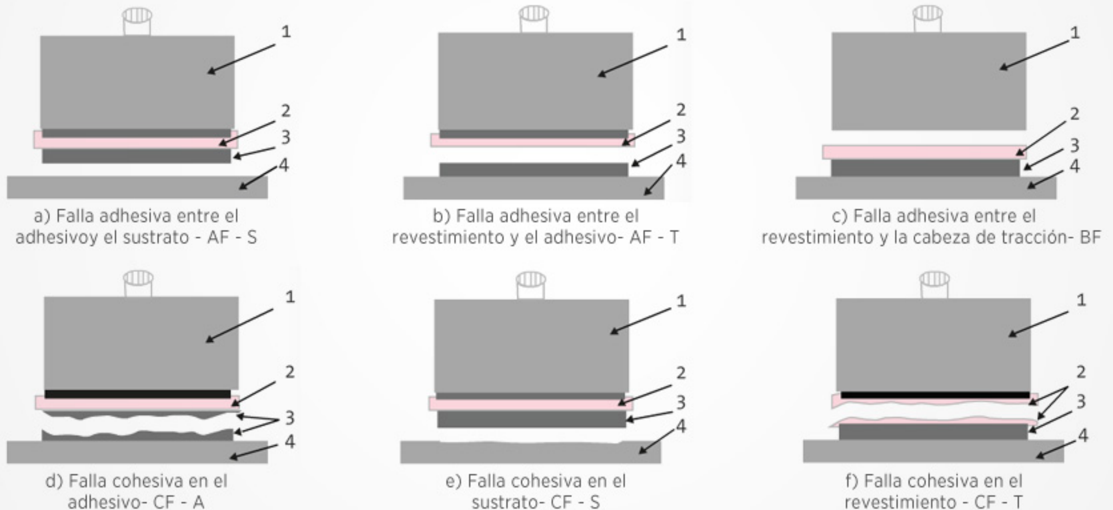
Figura 8-22: Tipos de falla de un sistema de revestimiento, según ISO 13007. (Adaptada de ISO 13007-2011)
